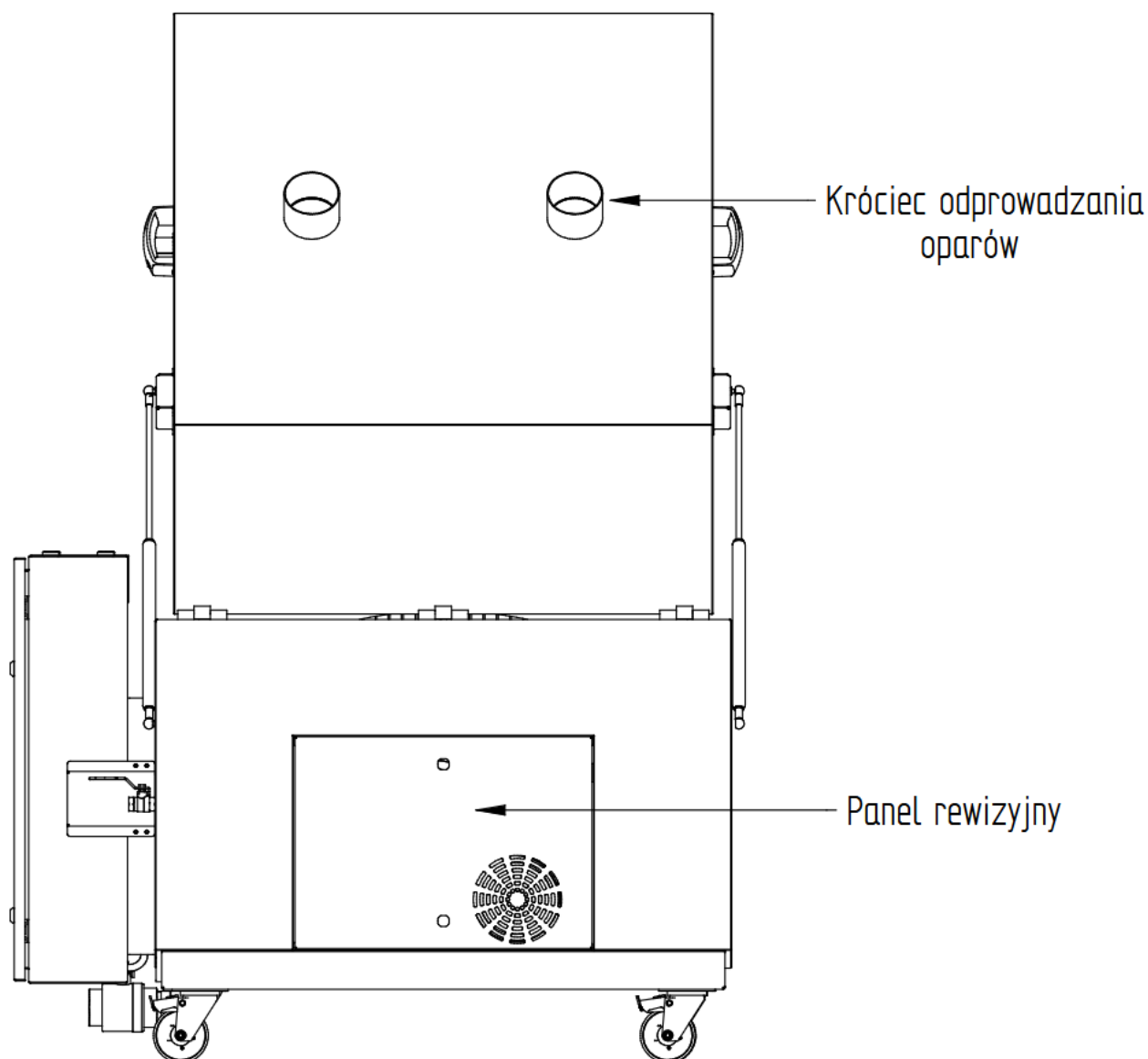
Rysunek 3 Widok ogólny z tyłu
