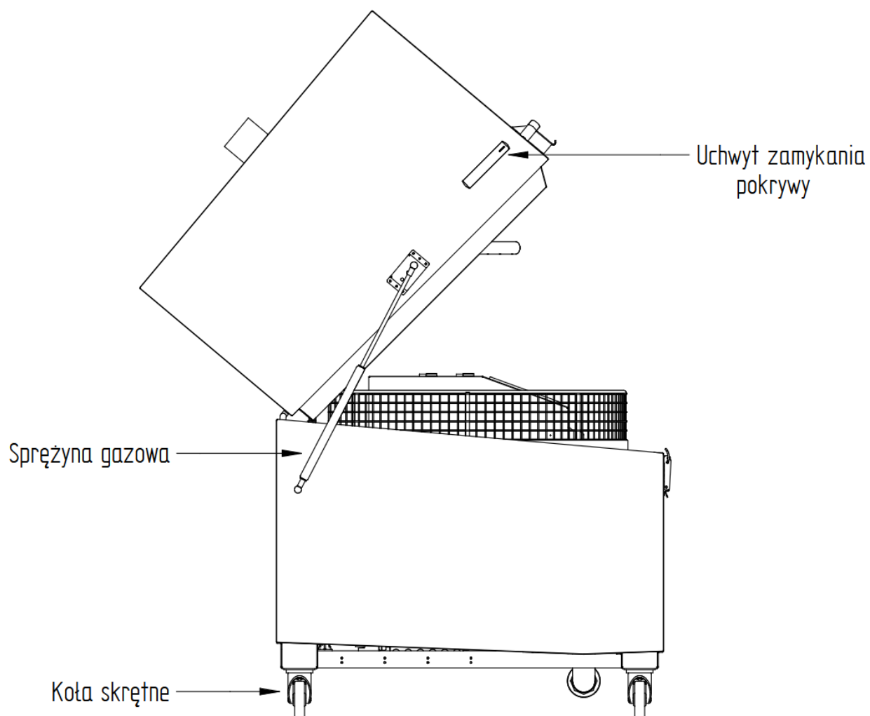
Rysunek 5 Widok ogólny z lewego boku
