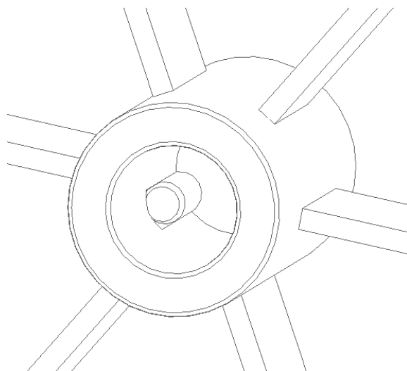
Rysunek 8 Widok umiejscowienia elementu zrywalnego kosza
