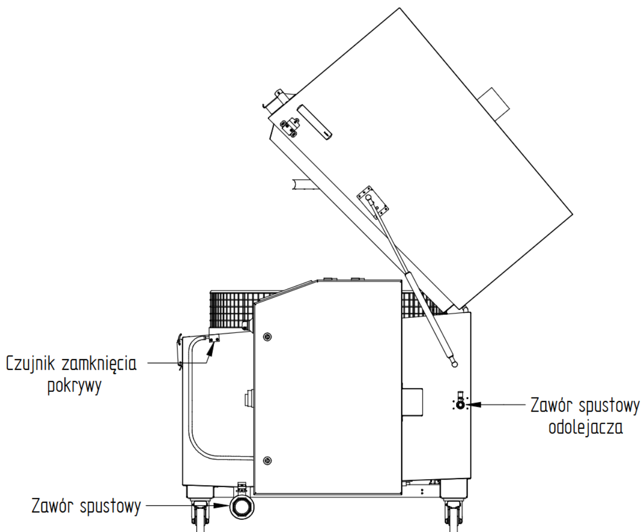
Rysunek 4 Widok ogólny z prawego boku
