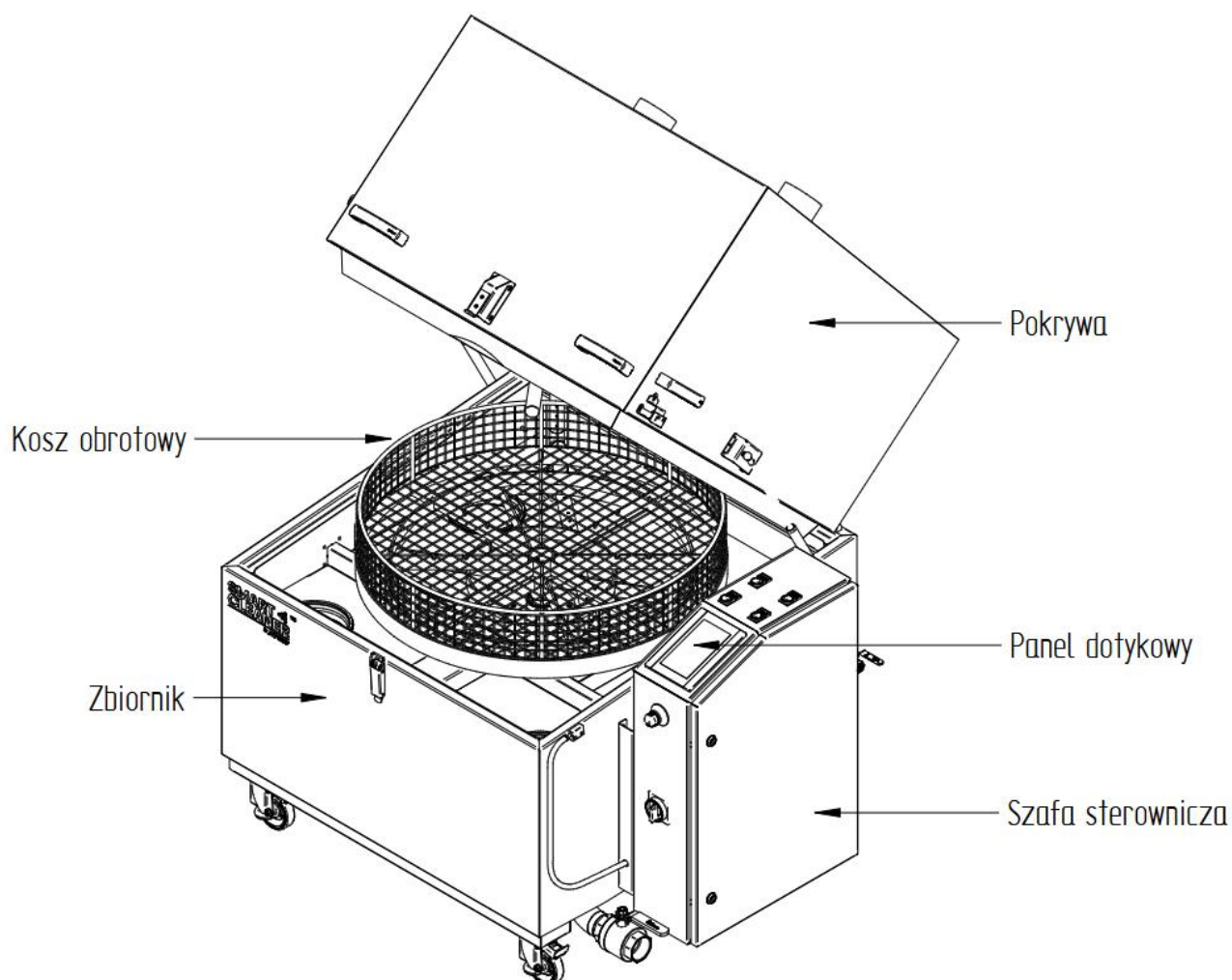
Rysunek 1 Rzut izometryczny
