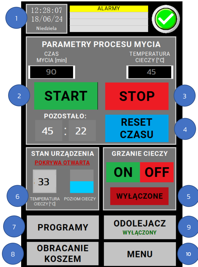
Rysunek 7 Widok Panelu dotykowego
