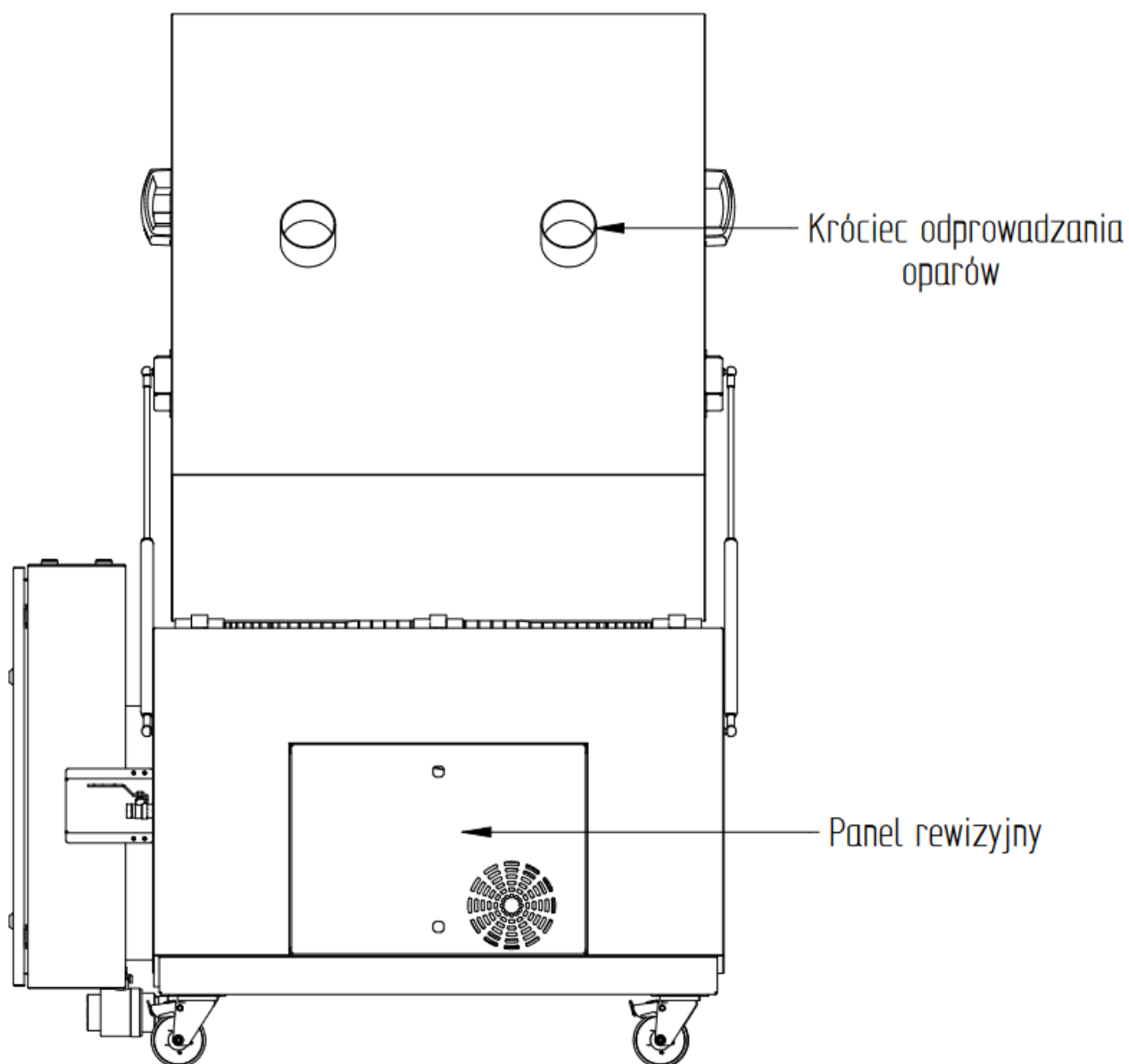
Rysunek 3. Widok ogólny z tyłu
