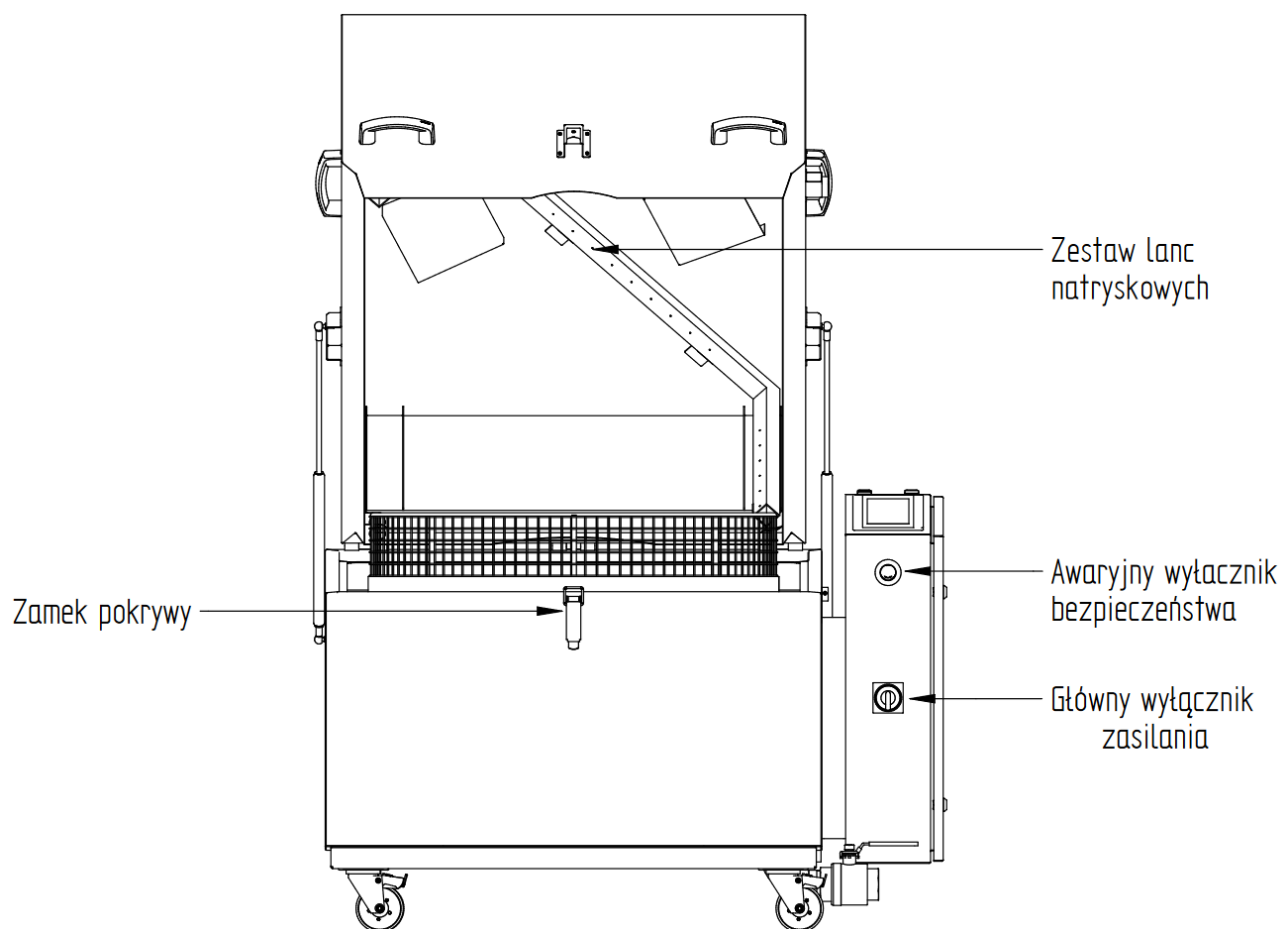
Rysunek 2. Widok ogólny z przodu
