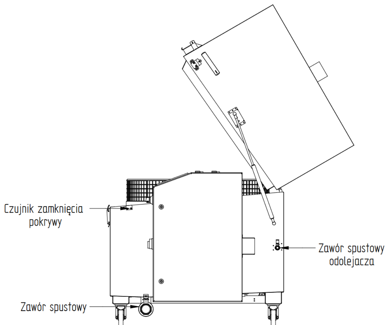
Rysunek 4. Widok ogólny z prawego boku
